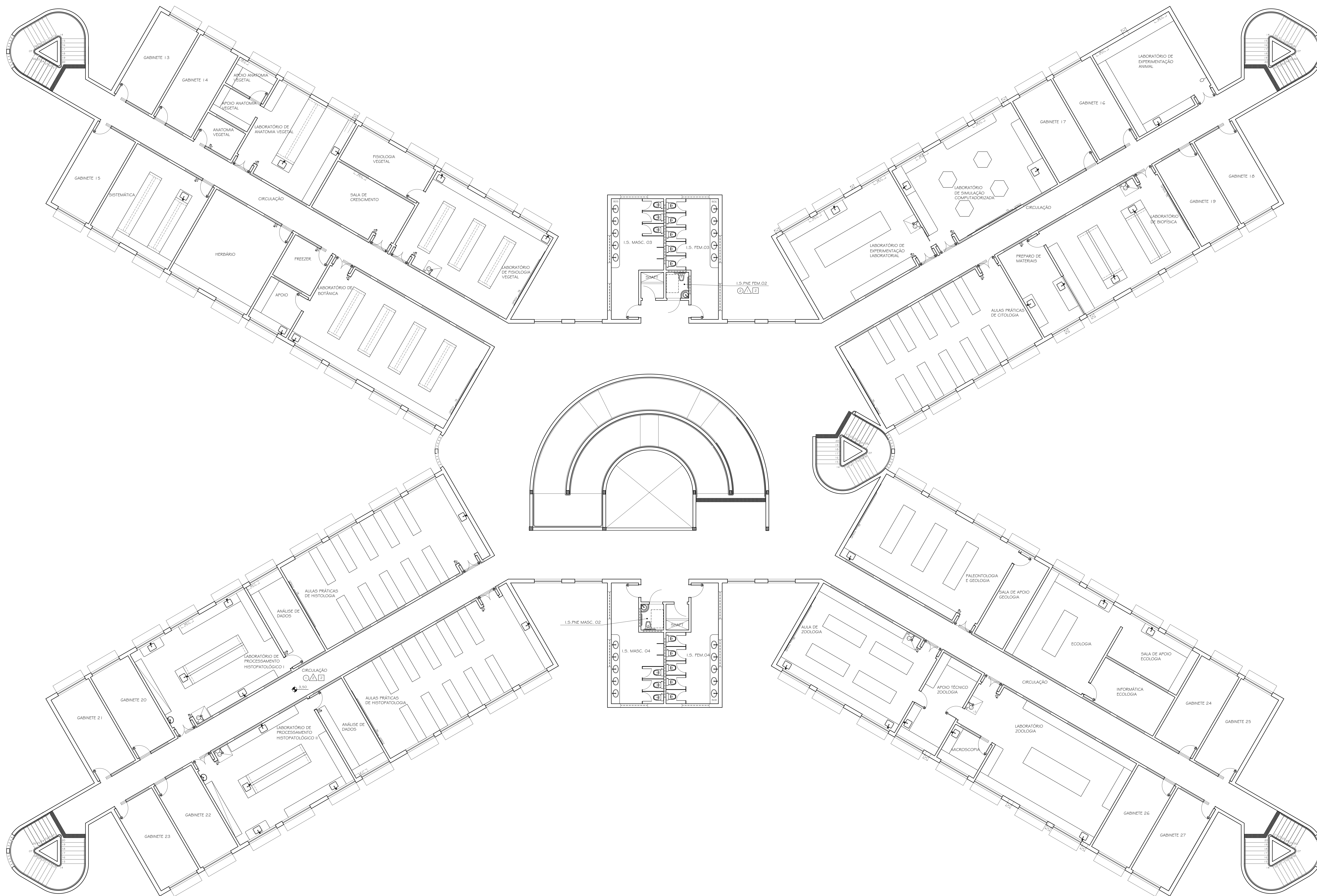
PLANTA 2º PAVIMENTO - PRÉDIO FCBS
