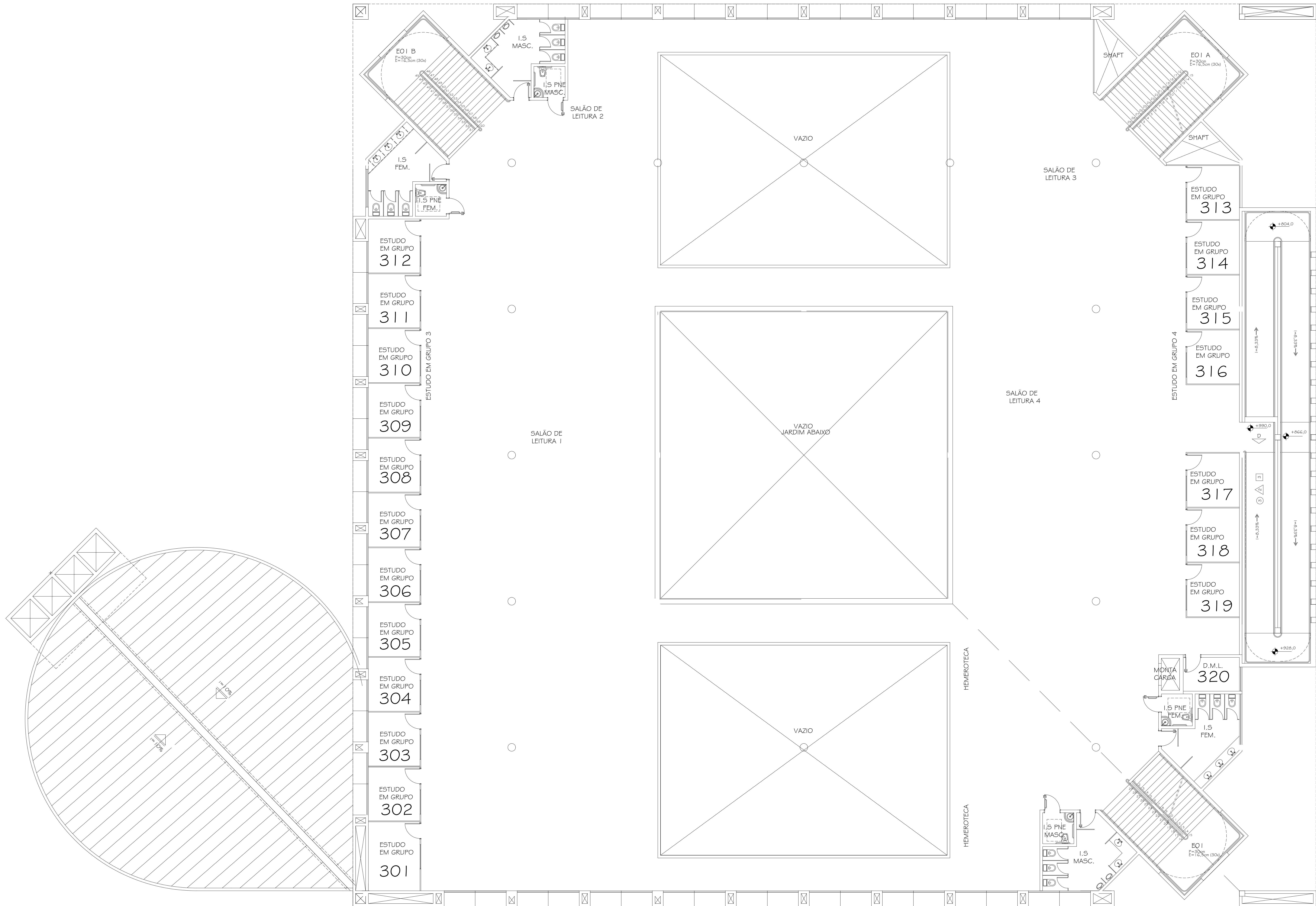
PLANTA LAYOUT 3º PAVIMENTO
