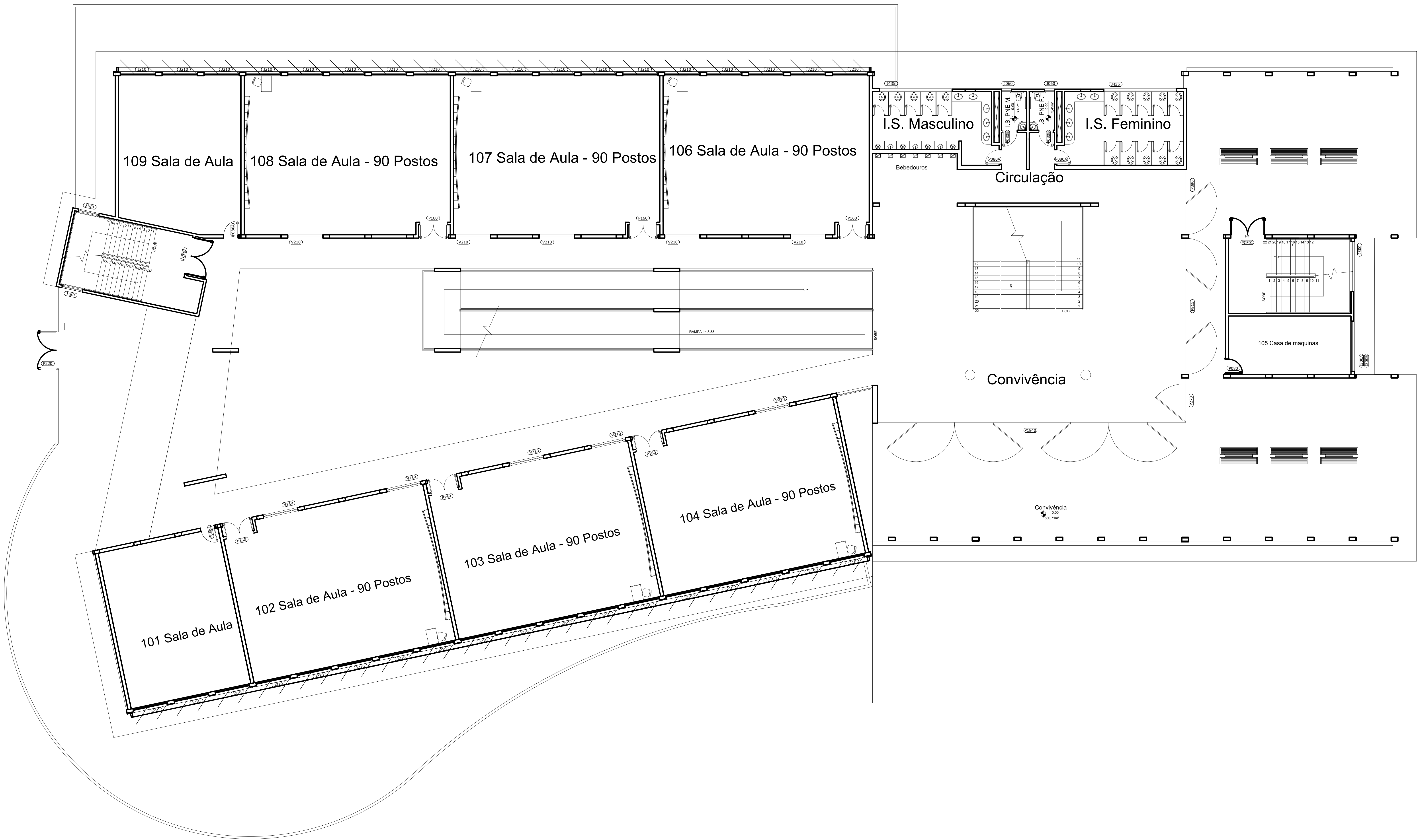
PLANTA DO TÉRREO - DETALHAMENTO DE ESQUADRIAS
