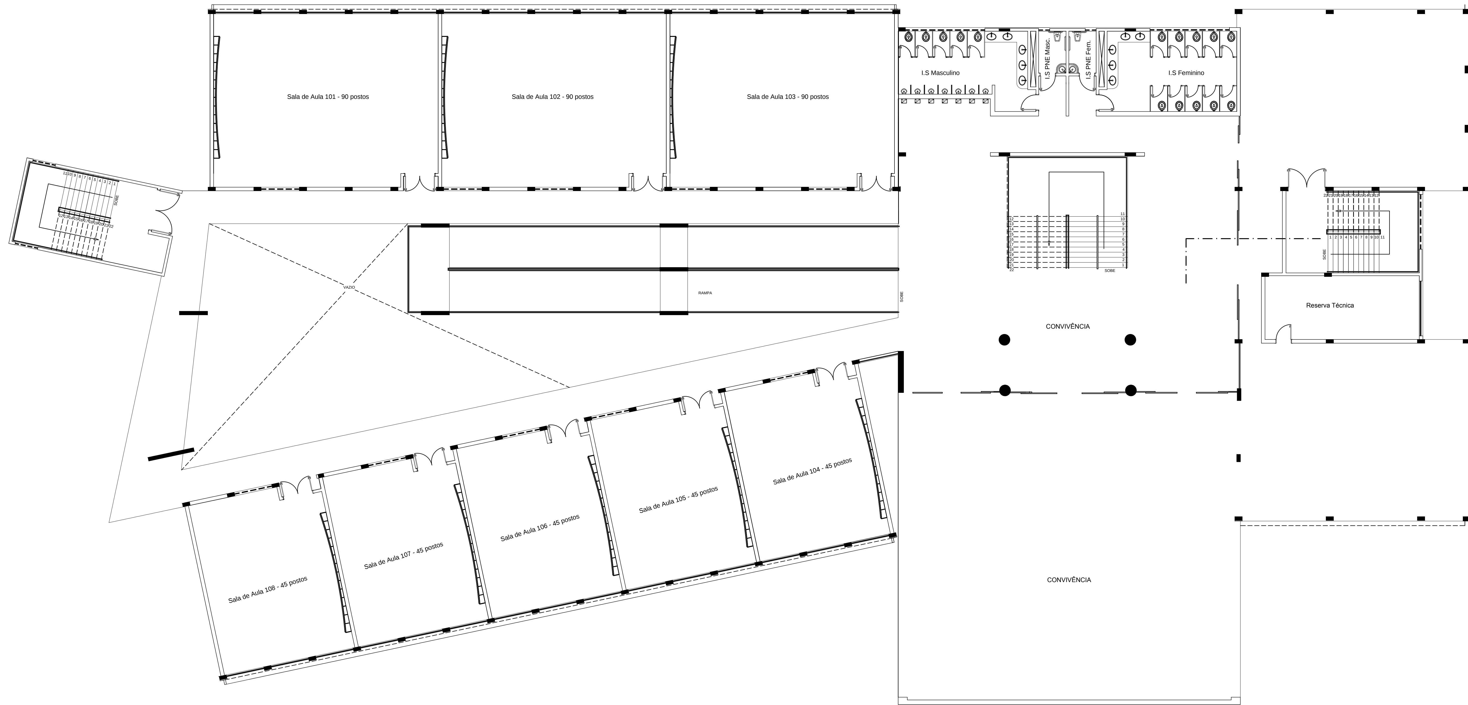
planta baixa - pavto térreo escala 1/100
