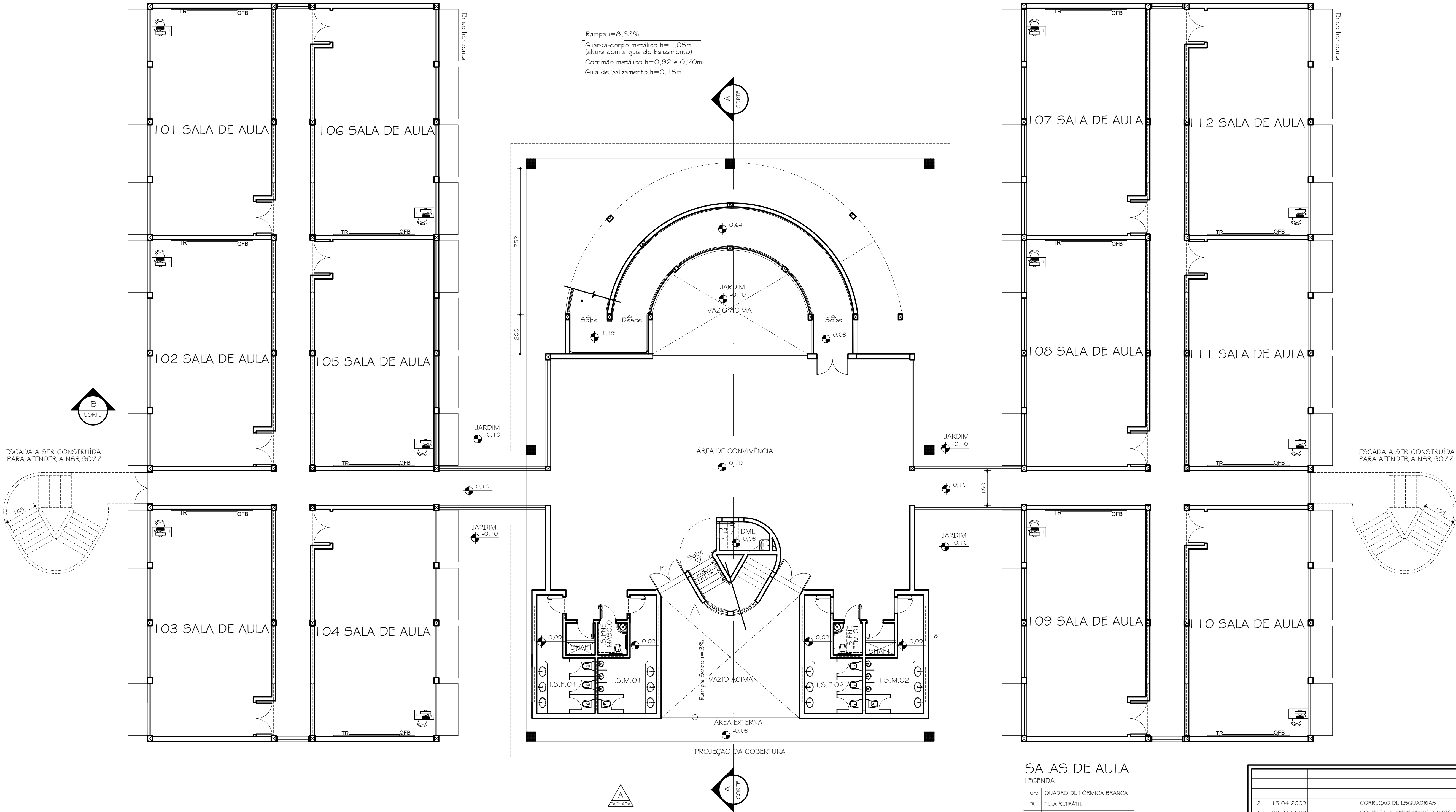
PLANTA 1º PAVIMENTO ESC. 1:100
