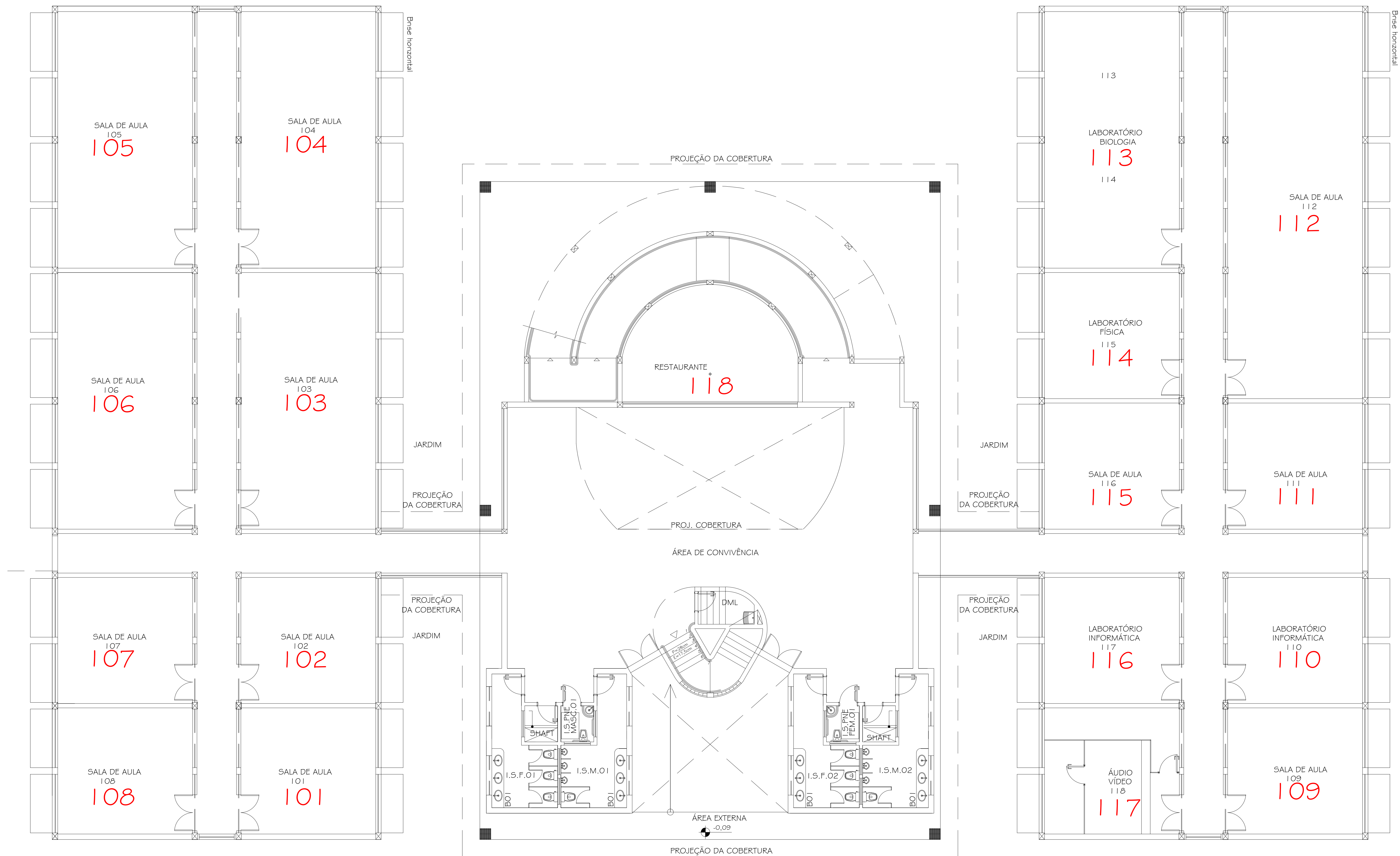
PRÉDIO DE AULAS PLANTA 1º PAVIMENTO
