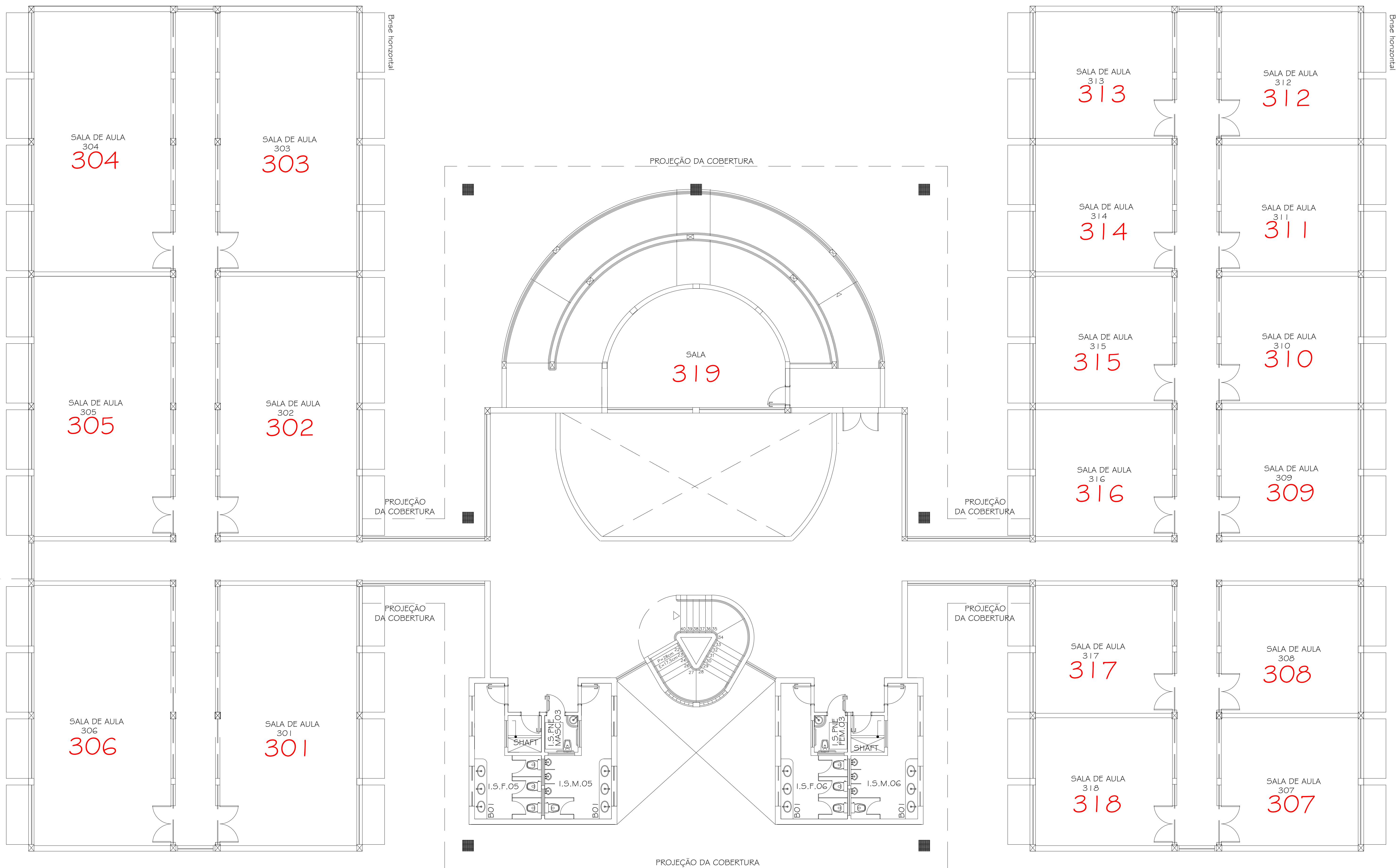
PRÉDIO DE AULAS PLANTA 3º PAVIMENTO
