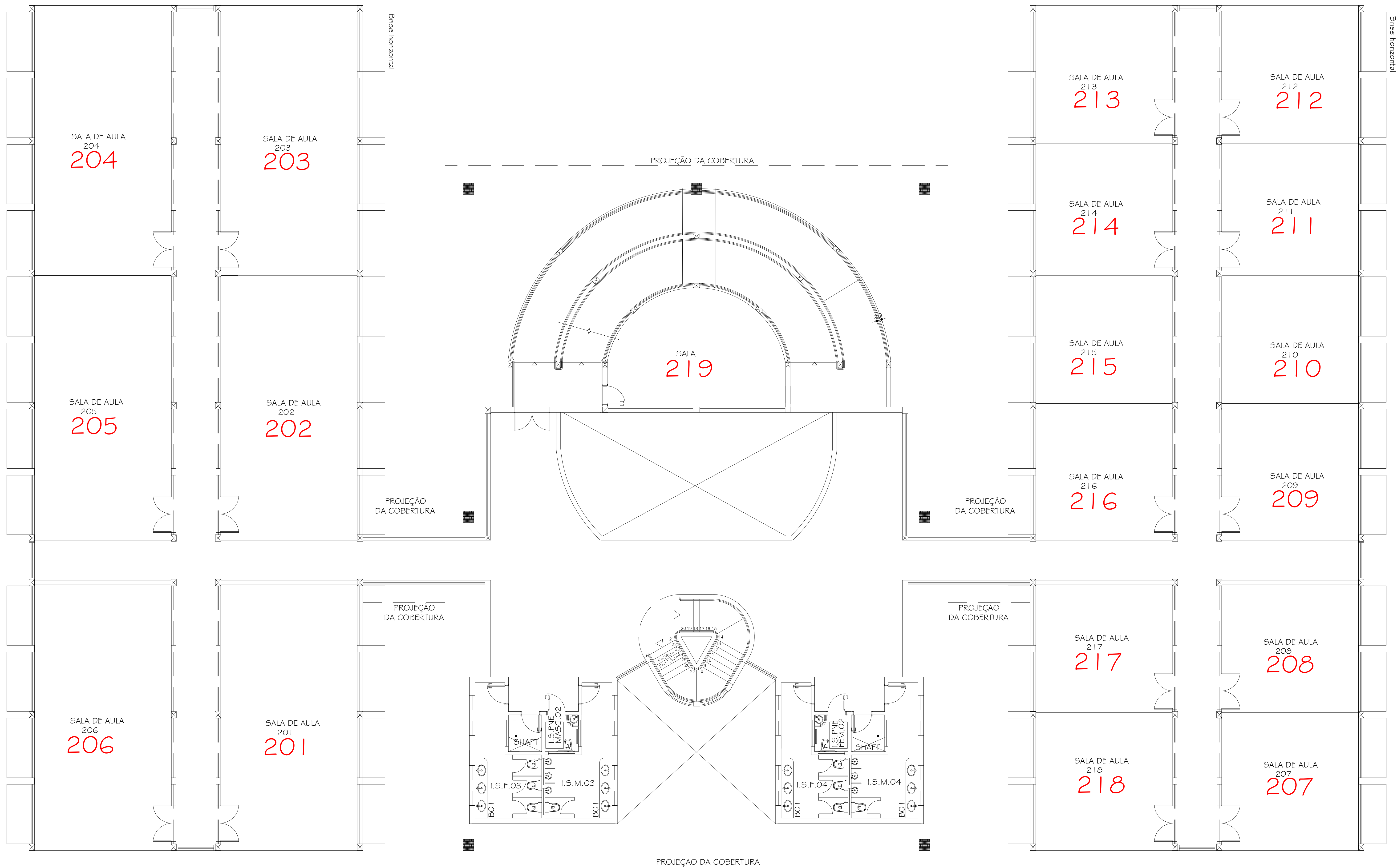
PRÉDIO DE AULAS PLANTA 2º PAVIMENTO
